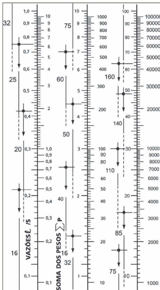
Diâmetros de Tubos de PVC rígido e vazões em função da soma dos pesos
