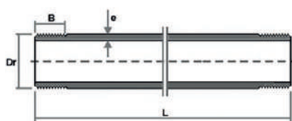
Dimensões (mm)
