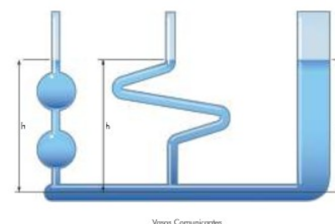
Vasos Comunicantes
