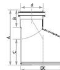
Redução Excêntrica Esgoto SN
