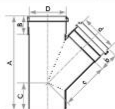
Junção Simples Esgoto SN
