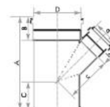
Junção com Redução Esgoto SN
