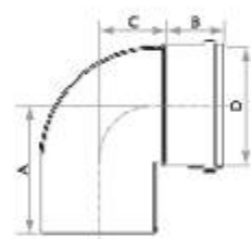
Joelho 90° Esgoto SN
