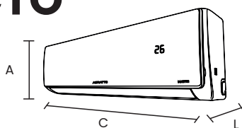
9K Btus - INT. (CxLxA) 770X250X201mm
